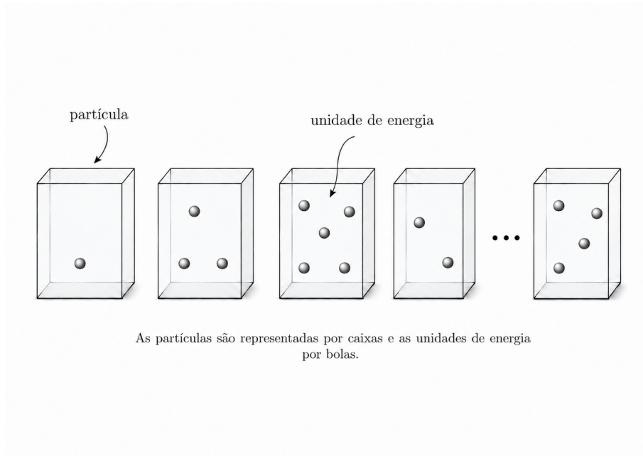
Figure 15: Representação esquemática do sistema constituído por partículas e unidades de energia.
