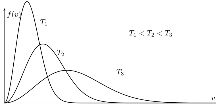
Figure 13: Representação qualitativa da distribuição do módulo das velocidades para diferentes temperaturas.
