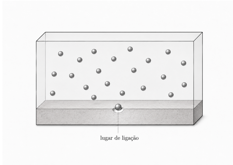
Figure 17: Representação esquemática de um sistema simples que obedece à distribuição grande canónica.
